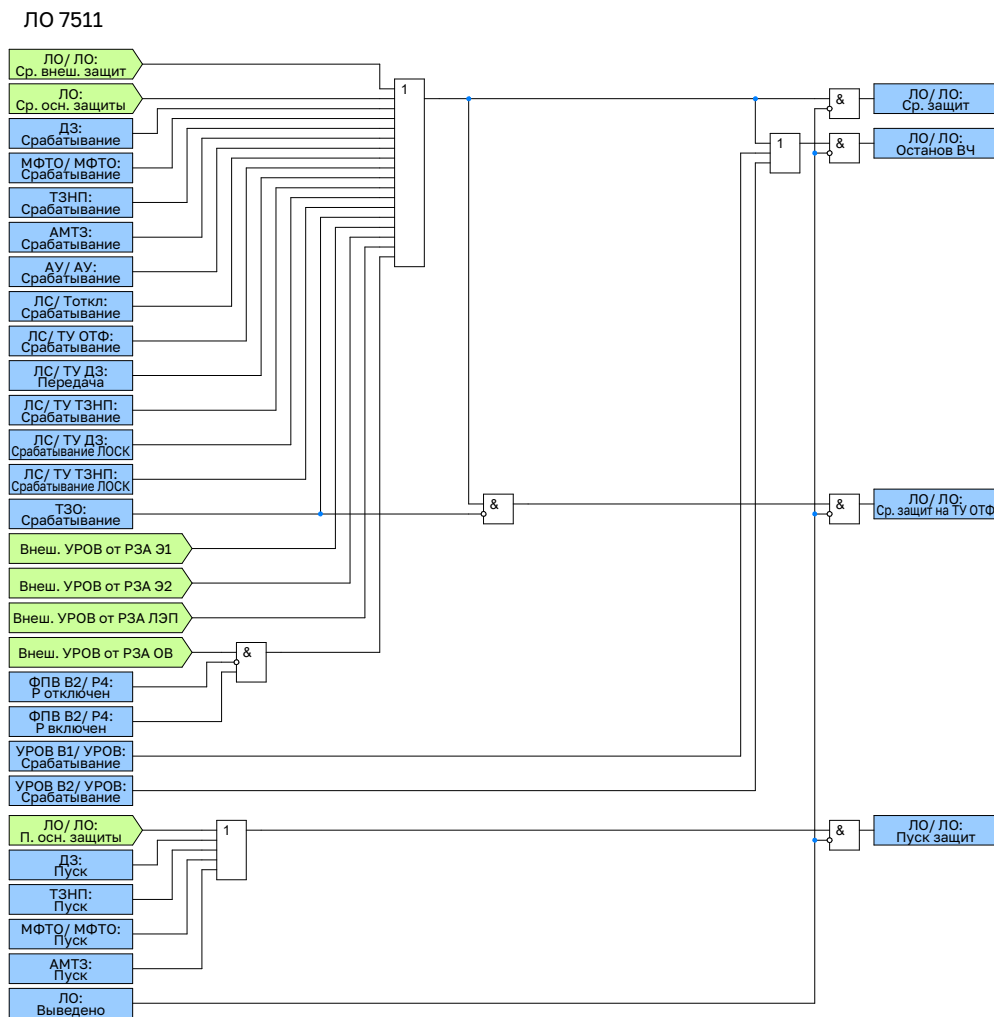
Рисунок 2.56 – Функциональная схема общей логики отключения
